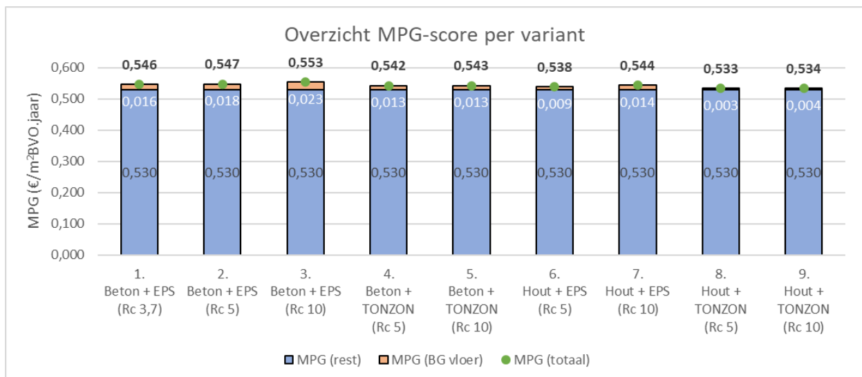
Figuur 3. Overzicht van MPG-scores (totaal en BG vloer) per variant.
