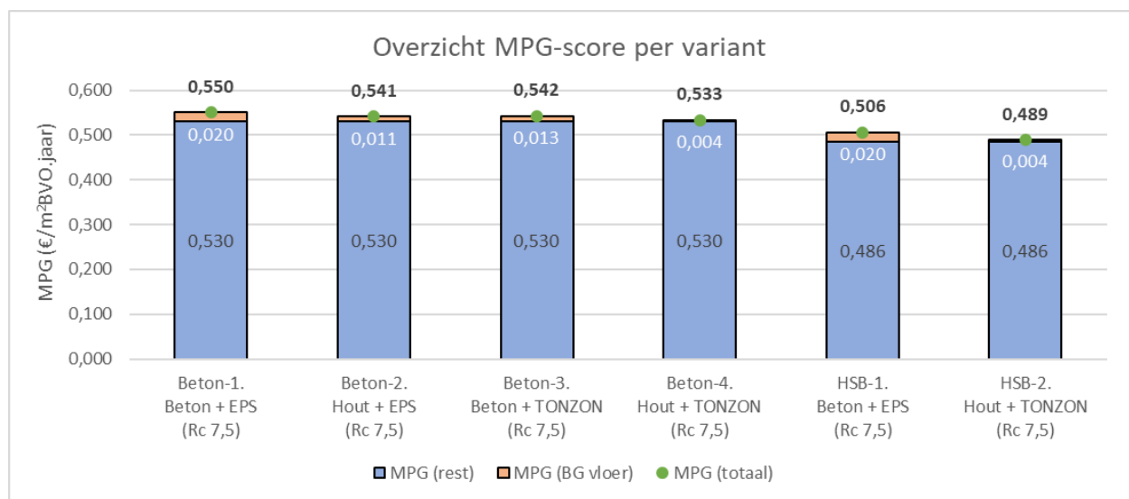
Figuur 5. Overzicht van MPG-scores (totaal en BG vloer) per variant.
