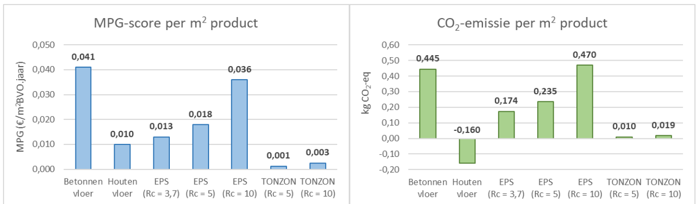
Figuur 2. MPG-score (links) en CO 2 -emissie (rechts) per m 2 materiaal op 1 m 2 BVO.
