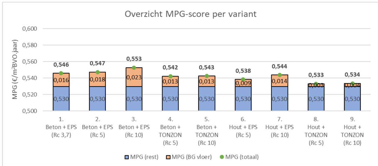
Figuur 4. Overzicht van MPG-scores (totaal en BG vloer) per variant, aangepaste schaal.
